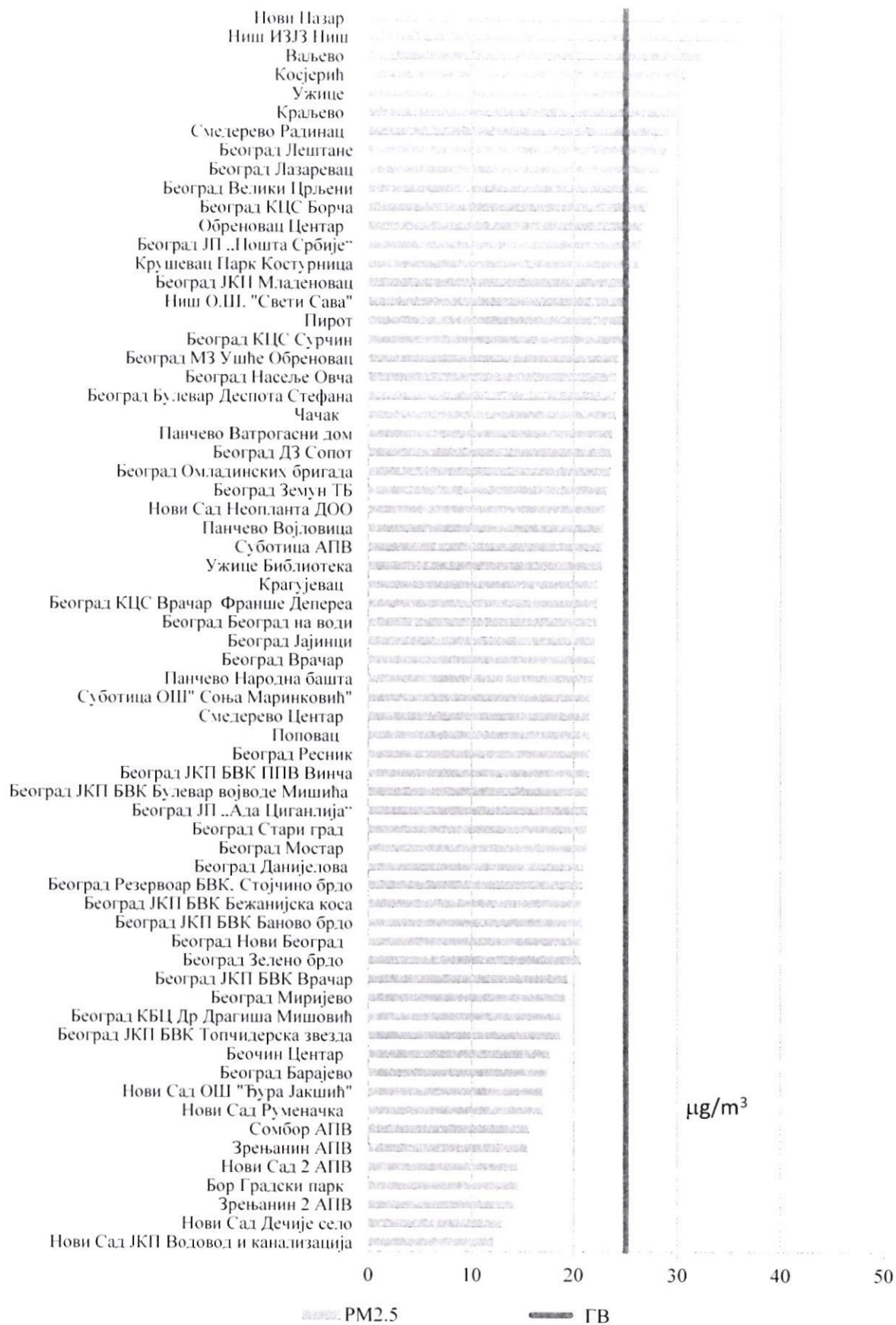
Слика 18. Средња годишња вредност концентрација \text{PM}_{2.5} у 2024. години
