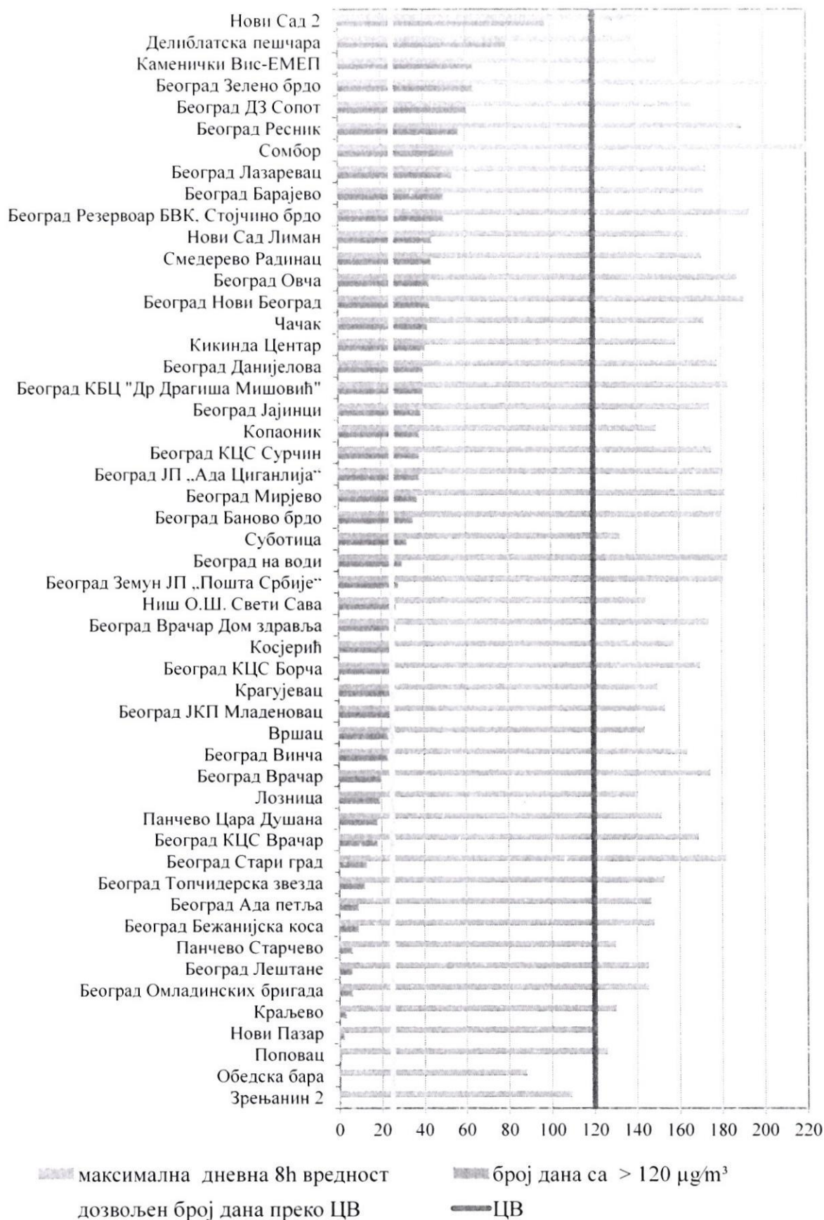
Слика 25. Упоредни приказ максималних дневних осмосатних концентрација O_3 ( \mu g/m^3 ) и броја дана са прекорачењем циљне вредности (у даљем тексту: ЦВ) у 2024. години
