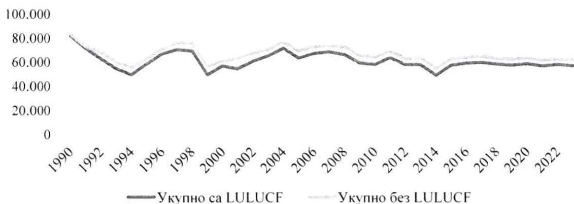
Слика 45. Укупне емисије гасова са ефектом стаклене баште (са и без LULUCF), CO 2 eq (kt)
