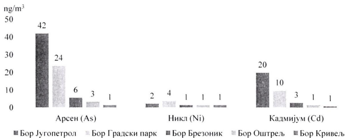
Слика 19. Средње годишње концентрације тешких метала (арсена, кадмијума и никла) у Бору у 2024. години
