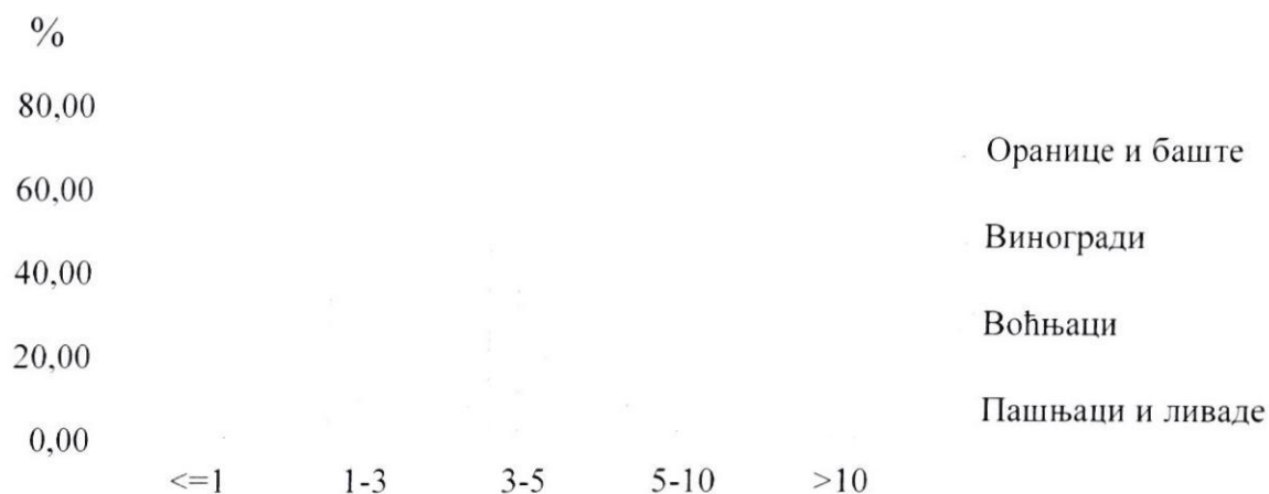
Слика 136. Садржај хумуса (%)
