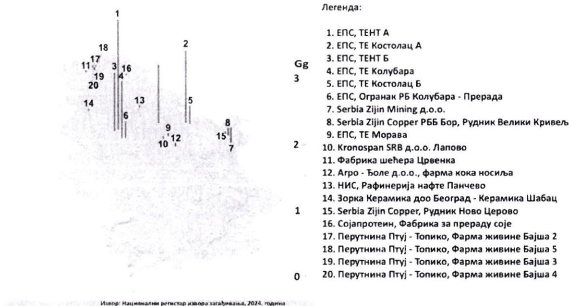
Слика 51. 20 најзначајнијих извора прашкастих материја у Републици Србији
