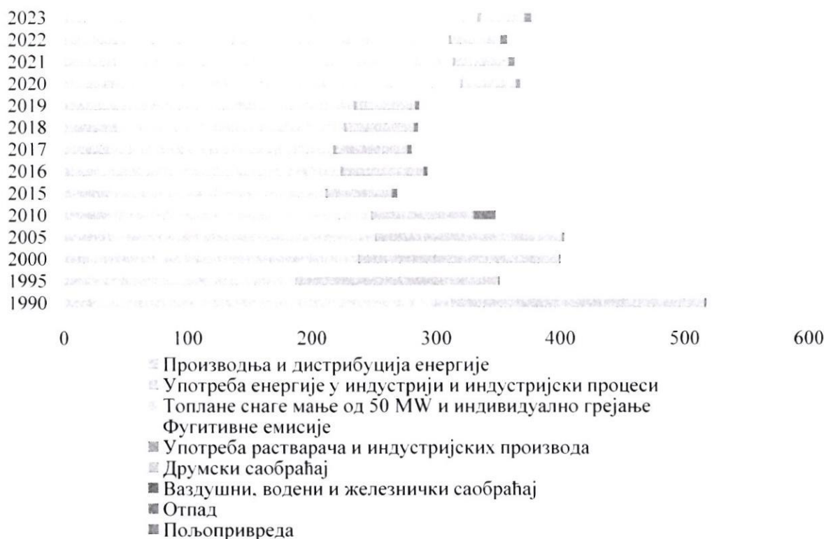
Слика 37. Емисија угљен-моноксида по секторима у периоду 1990-2023. година изражена у хиљадама тона
