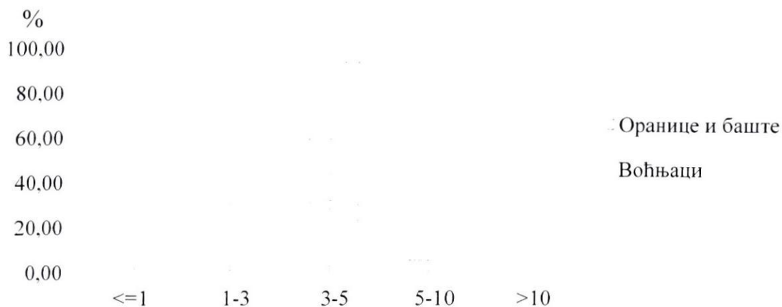
Слика 142. Садржај хумуса (%)
