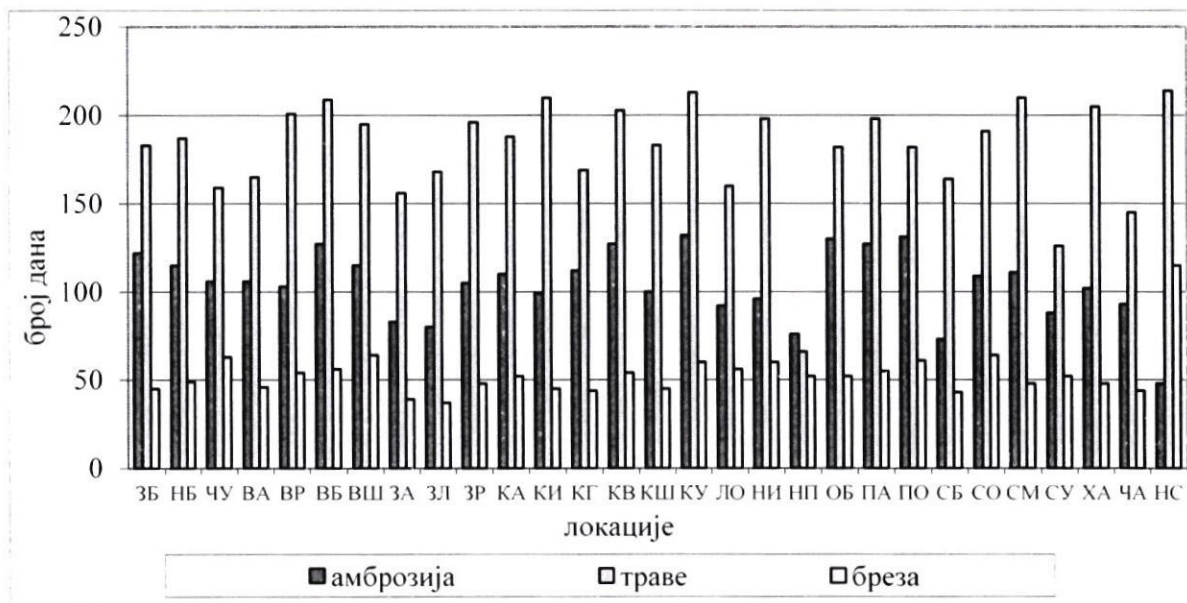
Слика 61. Број дана са присутном полинацијом за све станице у Републици Србији у 2024. години
