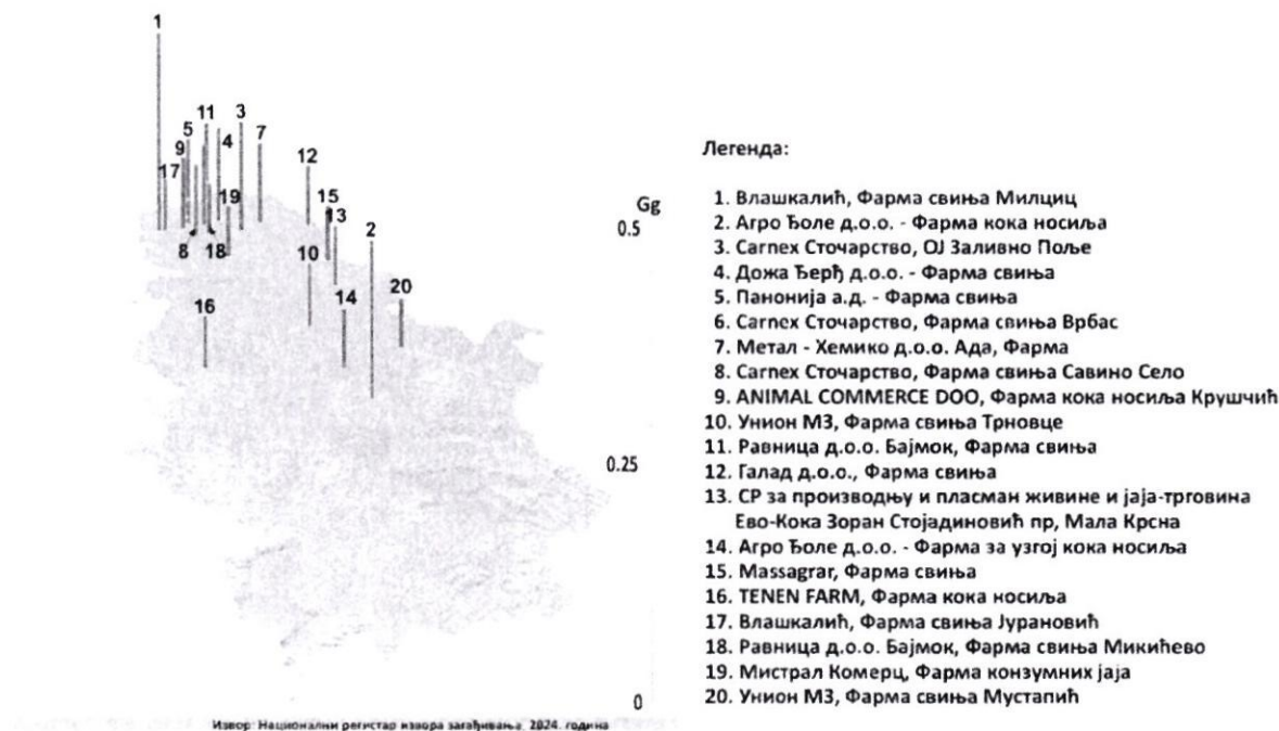
Слика 52. 20 најзначајнијих извора амонијака у Републици Србији
