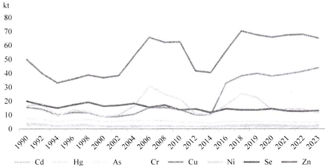
Слика 41. Емитоване количине Hg, Cd, As, Cu, Cr, Ni, Se, Zn у Републици Србији у периоду 1990-2023. године
